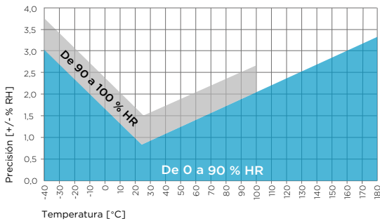
Precisión de HMP4 en la medición de humedad en función de la temperatura
