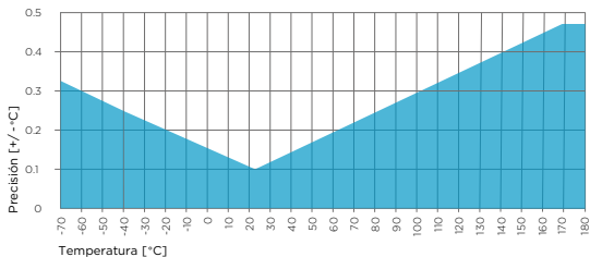
Precisión de HMP4 en la medición de temperatura sobre el rango completo
