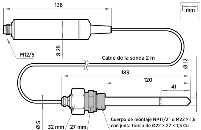
Dimensiones de la sonda HMP4
