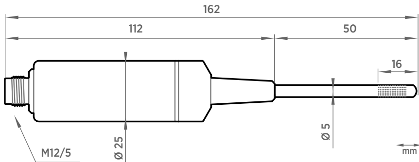
図 25 HMP1 プローブの寸法
